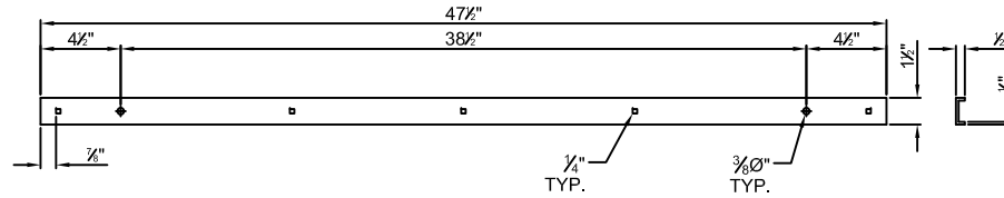
1 L-11 STIFFENER/GRIPPER DETAIL SCALE: NA
