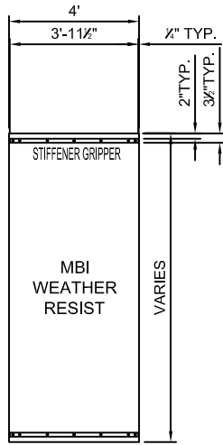
A L-11 STIFFENER/GRIPPER DETAIL SCALE: NA
