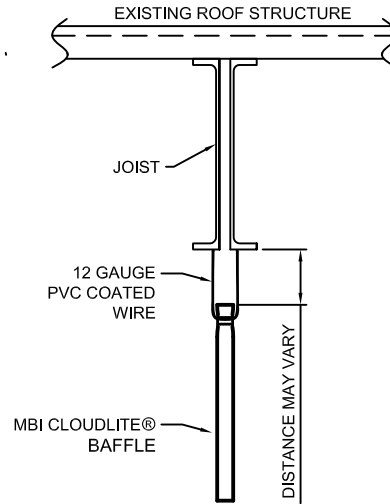
2 CL-03A SIDE ELEVATION SCALE: NA
