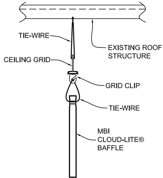
2 CL-04 SIDE ELEVATION SCALE: NA
